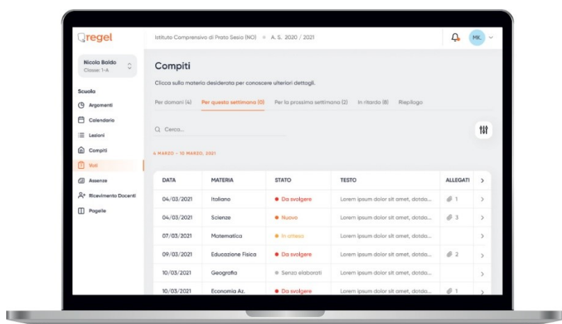
Interfaccia desktop
